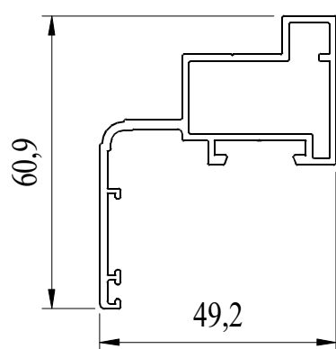
TS14 ościeżnica
