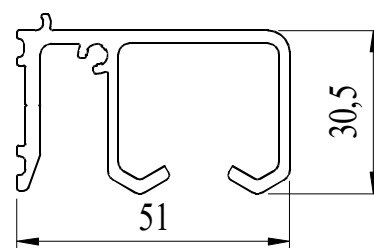
TS31 szyna
