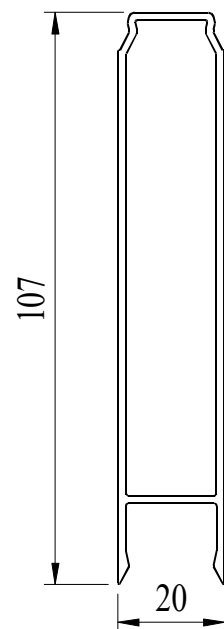
TS70 deska
