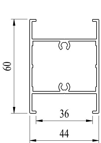
TS02 poprzeczka
