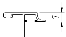
TS05 przymyk
